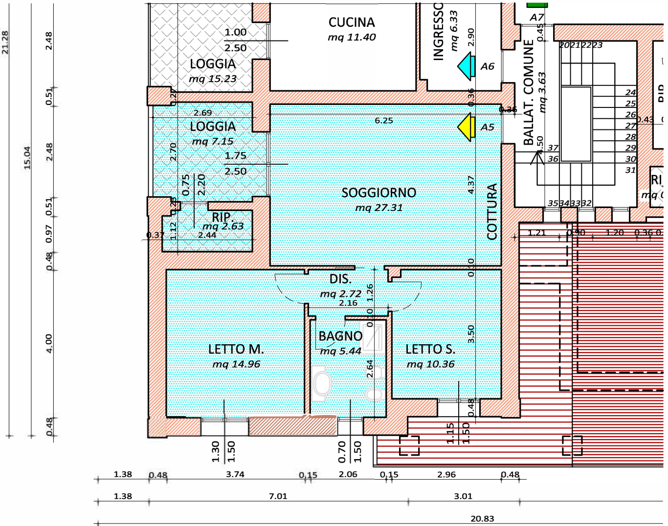
PIANO SECONDO SCALA 1:100
